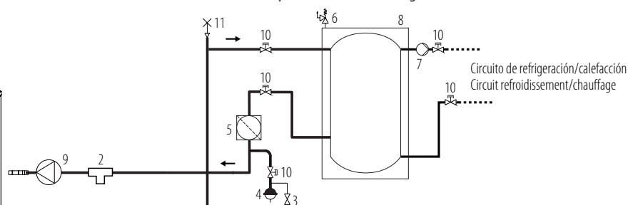
Pompe à chaleur avec configuration standard
