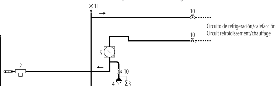
Pompe à chaleur avec configuration SI+PS/PSI/PD/PDI
